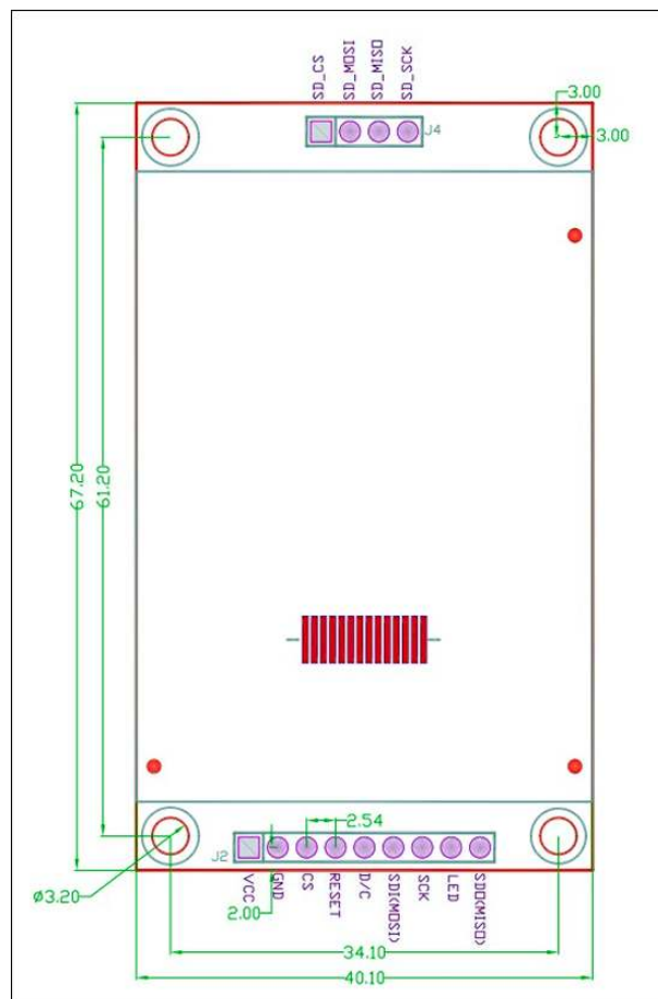
Рис.2 Установочные размеры
